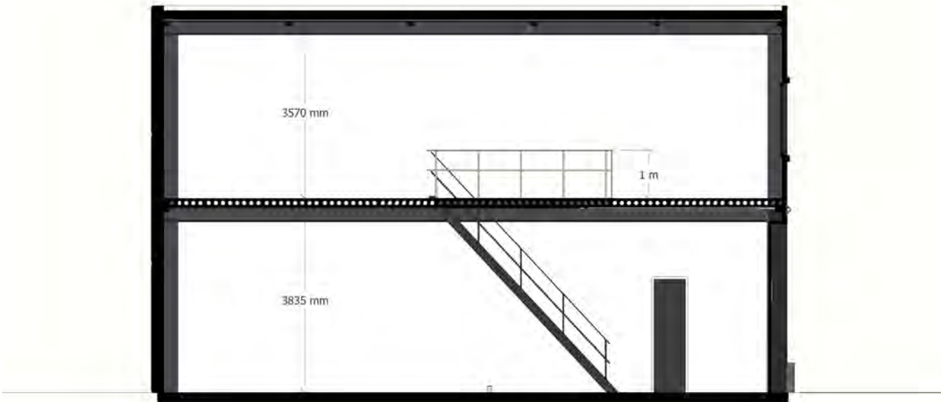
Doorsnede zijkant
